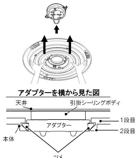
埋込引掛シーリングボディ
