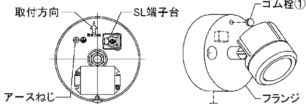
図-4 本体内面
