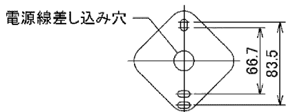
図-2 取り付け寸法図
