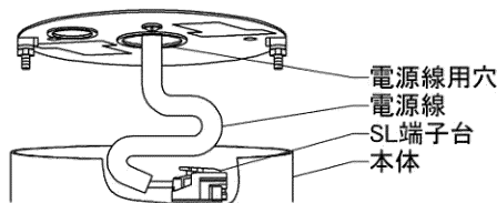
図-6 コード曲げ癖
