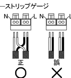
図-5 SL端子台
