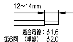
第6図（単線） 適合電線：φ1.6 φ2.0
