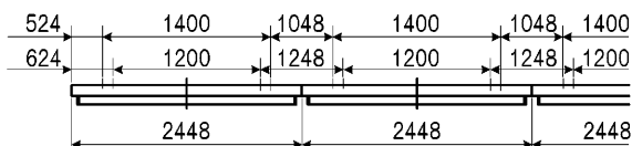
連結寸法図
