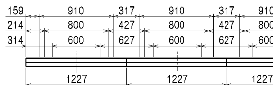
連結寸法図
