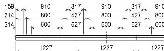
連結寸法図
