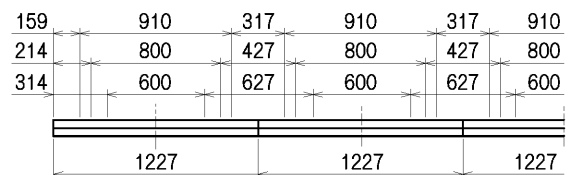
連結寸法図
