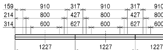
連結寸法図
