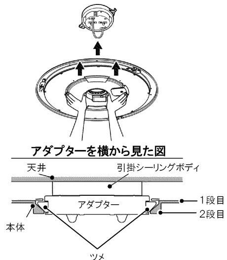
埋込引掛シーリングボディ
