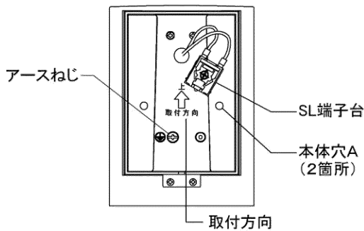
図-2 本体内部
