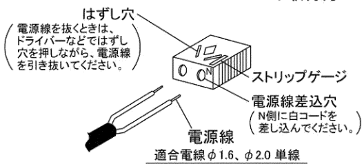
図-6 SL端子台
