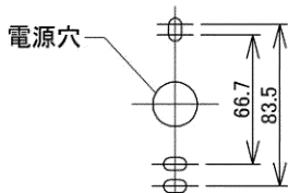
図-3 取付寸法図
