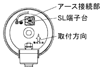
図-4 本体内部
