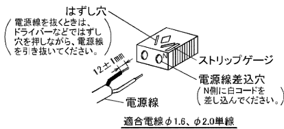
図-3 SL端子台
