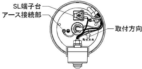
図-4 本体内部
