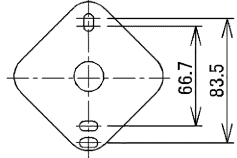
図-2 取り付け寸法図
