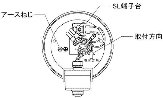
図-4 本体内面
