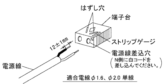
図-3 SL端子台
