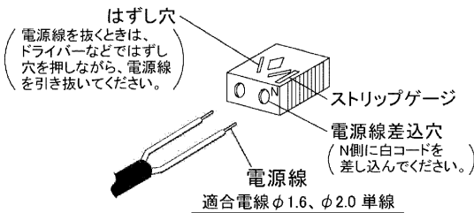
図-6 SL端子台
