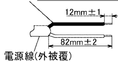
図-4 電源線皮むき寸法
