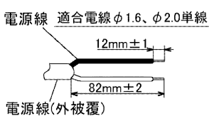
図-4 電源線皮むき寸法
