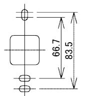
図-3 取り付け寸法図
