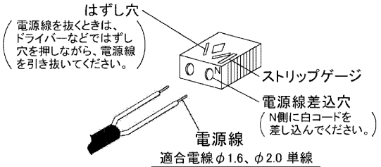
図-6 SL端子台
