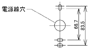
図-3 取付寸法図
