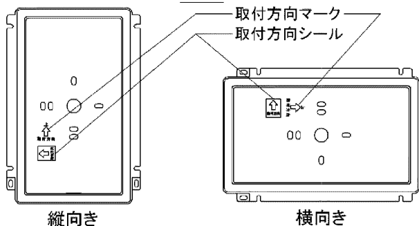
図-2 取付方向
