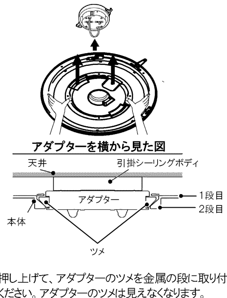
埋込引掛シーリングボディ
