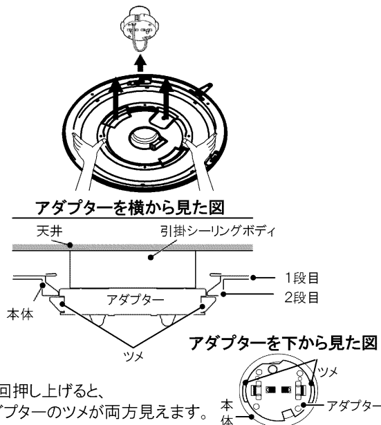
角形・丸形引掛シーリングボディ
