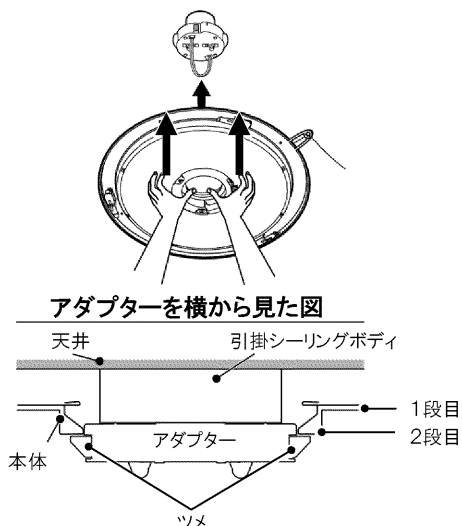
角形・丸形引掛シーリングボディ
