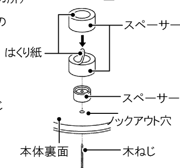
スペーサー (4個)
