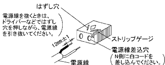
図-4 SL端子台
