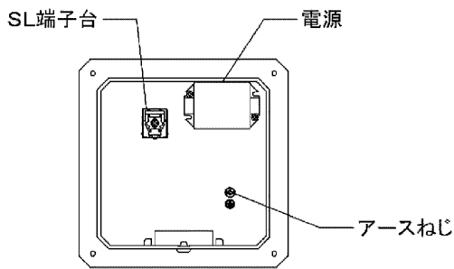
図-2 本体内部
