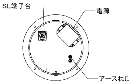
図-2 本体内部
