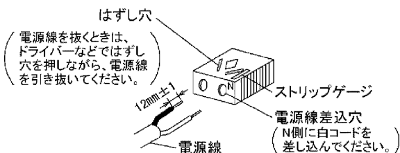
図-4 SL端子台
