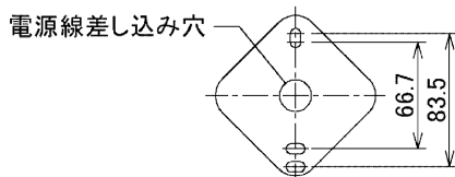
図-2 取り付け寸法図
