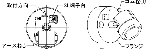
図-4 本体内面
