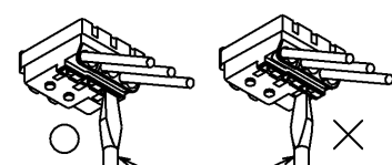
第3図 マイナスドライバー
