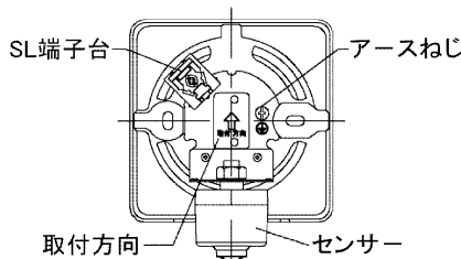
図-4 本体内部
