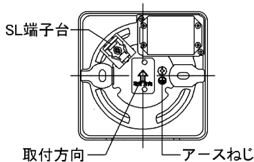
図-4 本体内部
