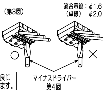
マイナスドライバー 第4図
