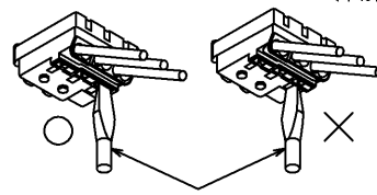
第3図 マイナスドライバー
