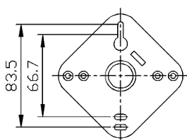
図-4 取り付け寸法図
