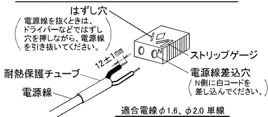
図-3 SL端子台
