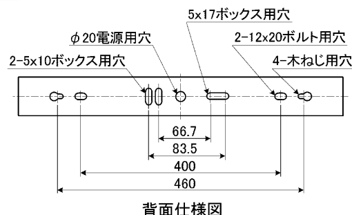
背面仕様図
