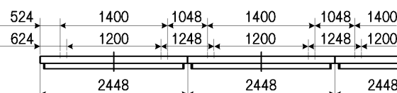
連結寸法図
