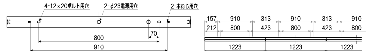
連結寸法図
