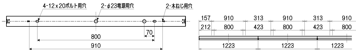
連結寸法図
