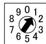
DF-70170-PD コントルク設定スイッチ図
