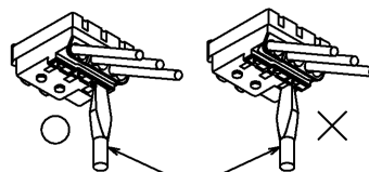
マイナスドライバー 第5図
