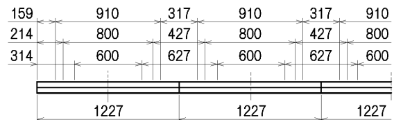
連結寸法図
