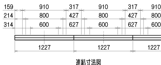
連結寸法図
