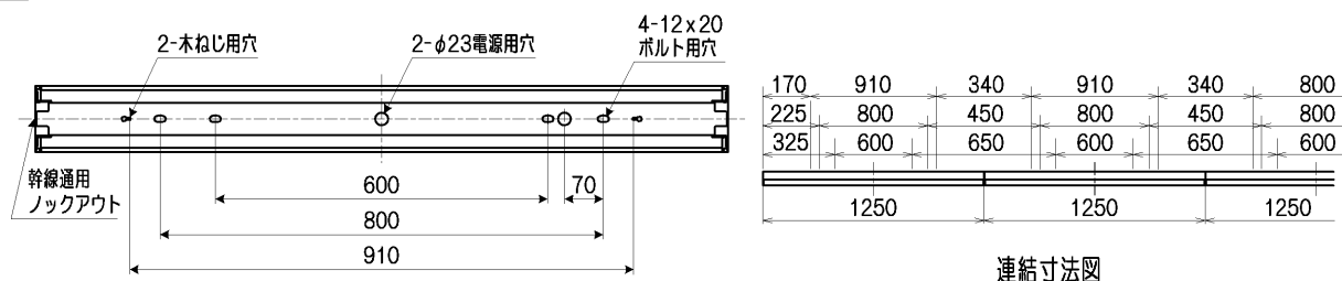
連結寸法図
