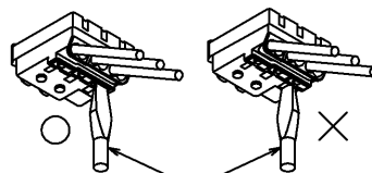
マイナスイドライバー 第6図
