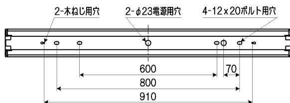
【LEET-40701-LS9】連結寸法図
