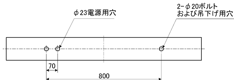
背面仕様図
