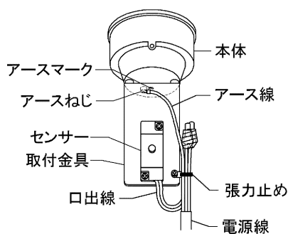
図-3 電源線の張力止め
