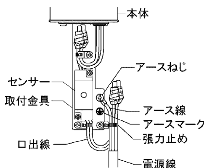
図-3 電源線の張力止め
