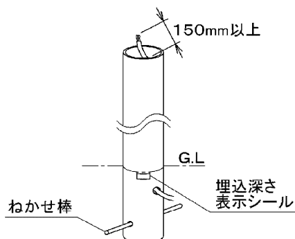
図-2 ポールの埋込み
