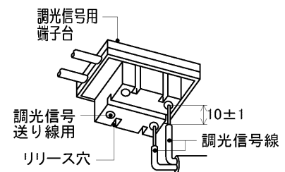
第5図 (適合電線 φ0.9, φ1.2 単線)
