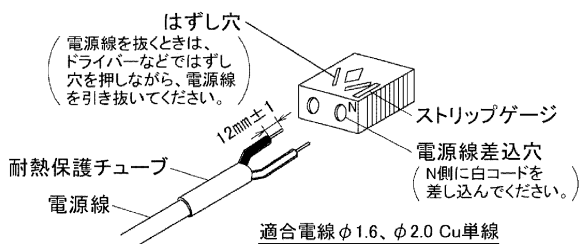
図-4 SL端子台
