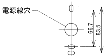
図-2 取り付け寸法図
