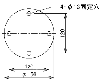
図-2 取り付け寸法図
