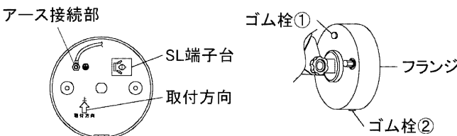
図-4 フランジ内面
