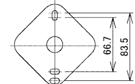
図-2 取り付け寸法図
