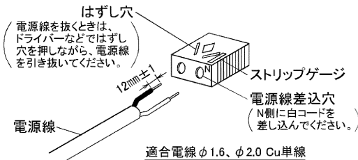
図-2 SL端子台
