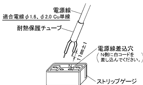
図-3 角形引掛シーリングボディ
